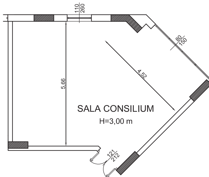
Pianta Piano 1 - scala 1:100 SALA CONSILIUM
